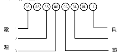
三相三線，直接型
