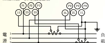
三相三線，併用變比器型
