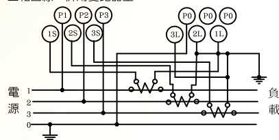
三相四線，併用變比器型
