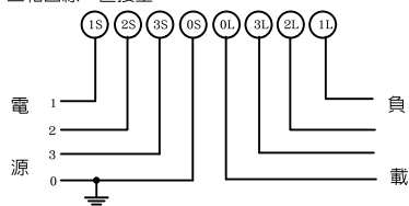
三相四線，直接型
