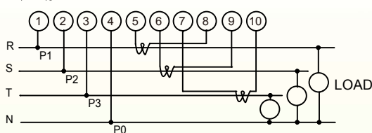
三相四線
