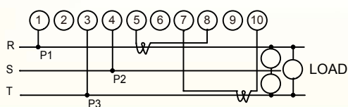
三相三線
